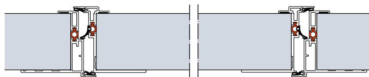
Конструкция калитки с термическим разделением для секционных ворот со строительной глубиной 67 мм
