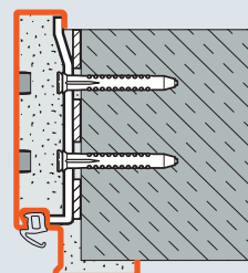
Dübelmontage durch die Zargenleibung (Sichtmauerwerk / Beton)
