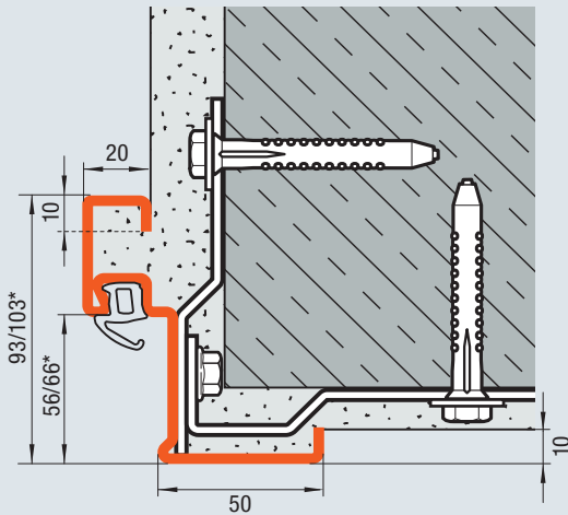
Dübelmontage (Mauerwerk / Beton)
