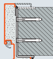
Schweißmontage (Porenbeton / Sichtmauerwerk)
